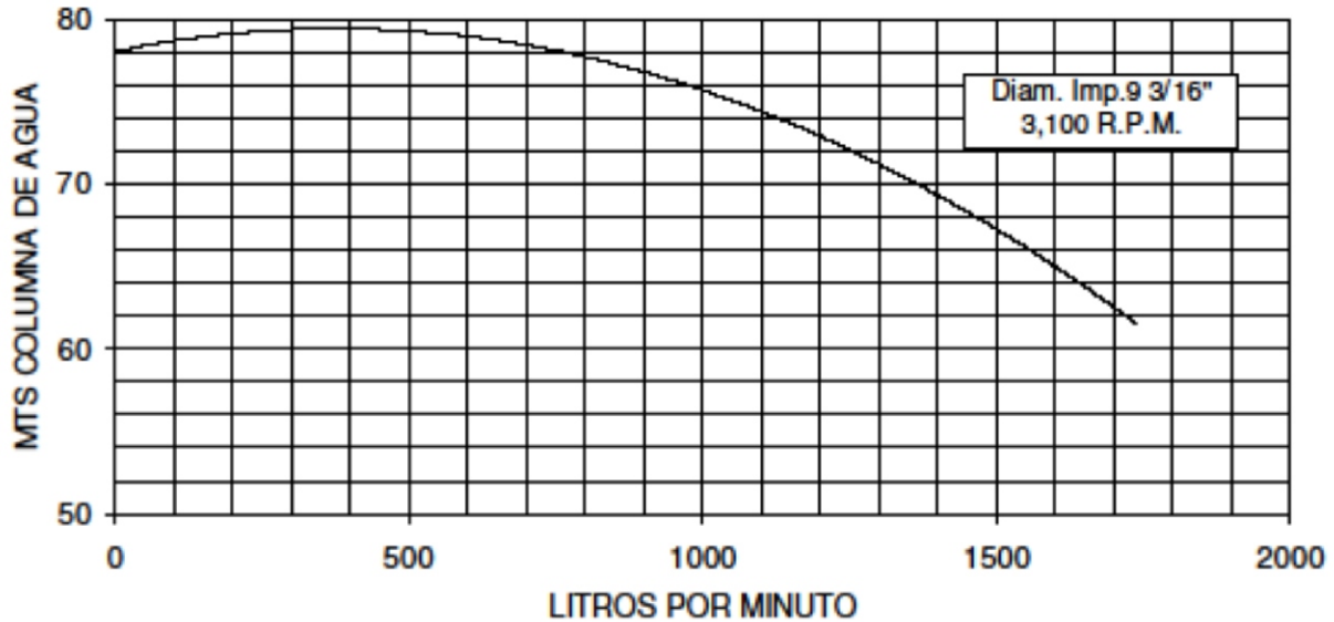
CURVA DE RENDIMIENTO CARGA-GASTO
