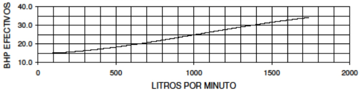
CURVA DE RENDIMIENTO GASTO-B.H.P.
